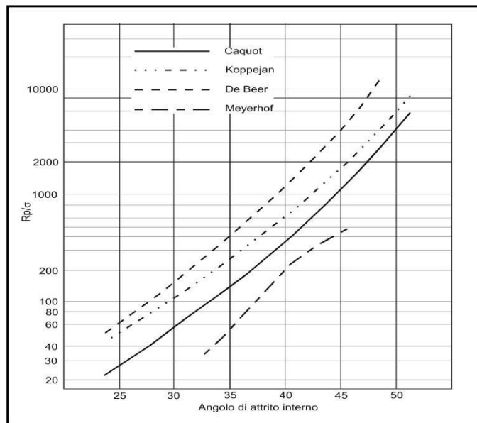
Fig. 14– Correlazione R_p - \phi
