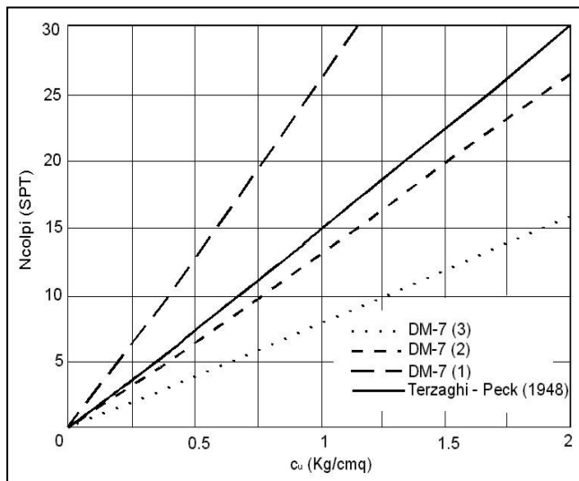
Fig. 12 - Correlazioni C_u - N_{SPT}
