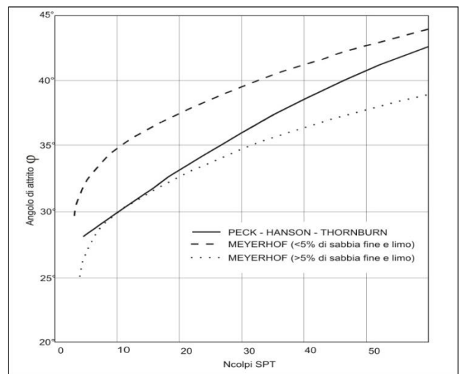
Fig. 13 - Correlazioni \phi - N_{SPT}
